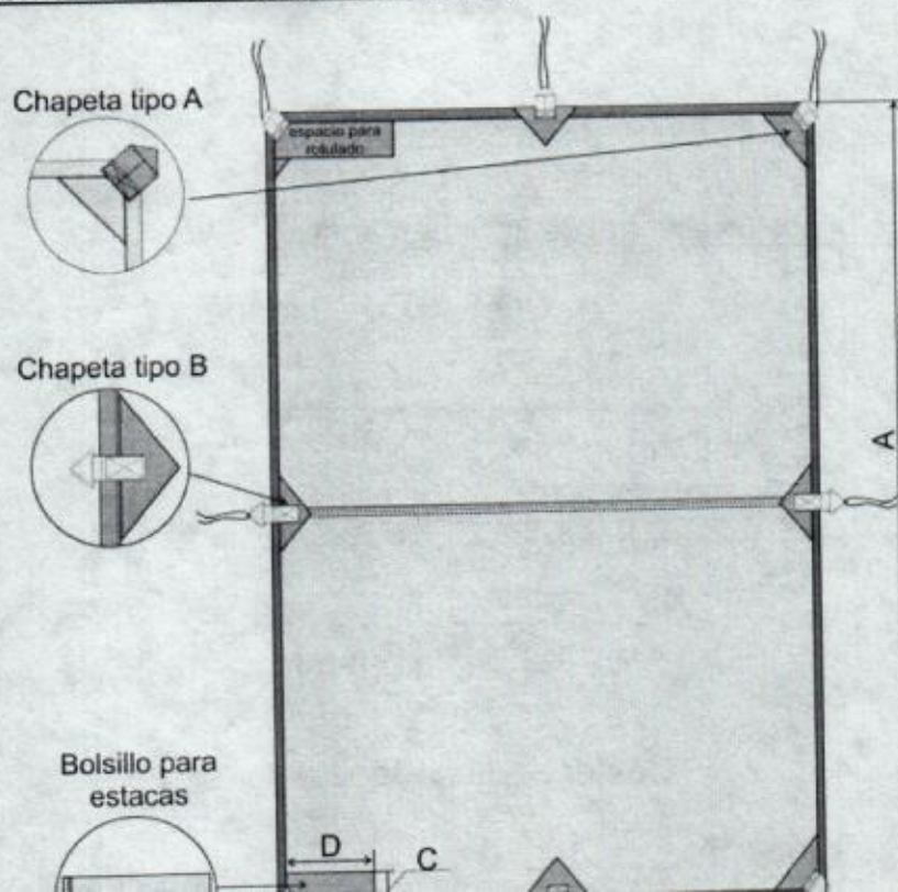
Figura 2. Vista interna de la Sobrecarpa extendida
