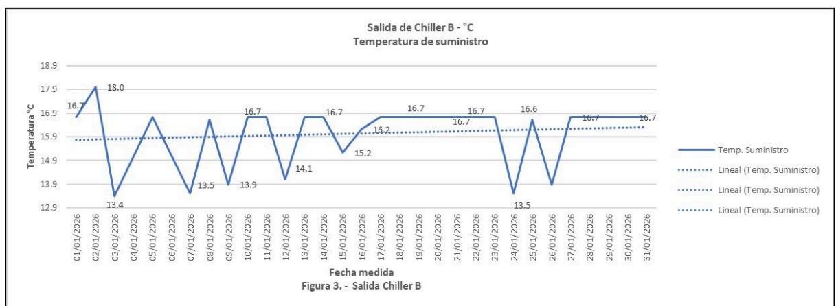
Figura 4 - Salida chiller B
