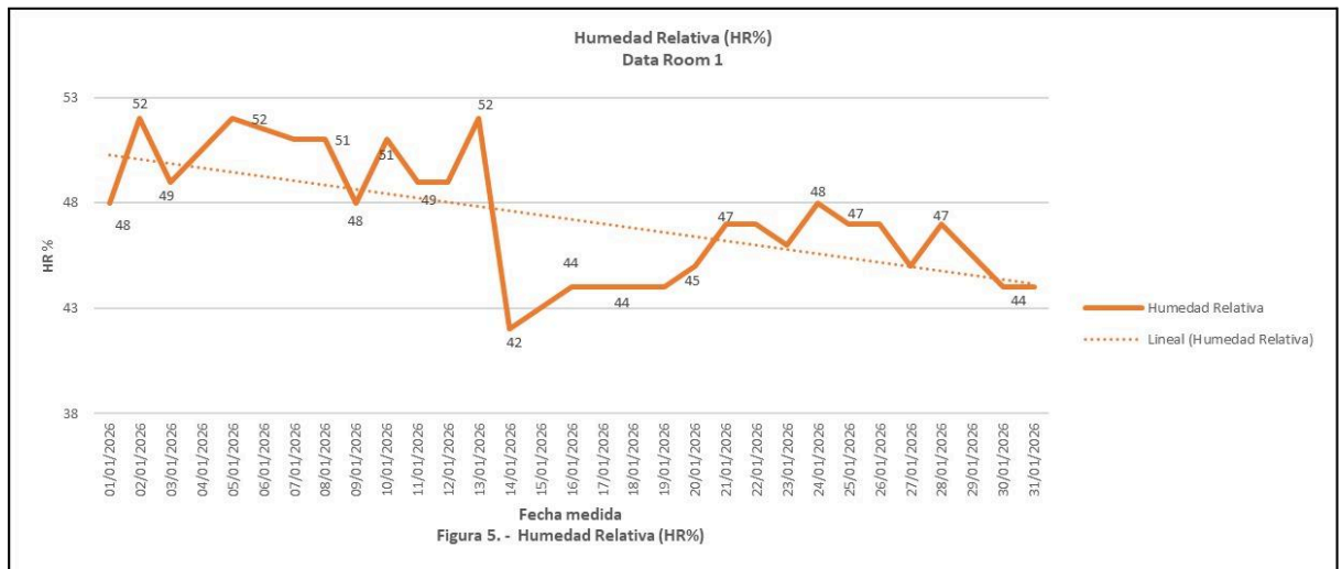
Figura 6 - Humedad Relativa (HR%)
