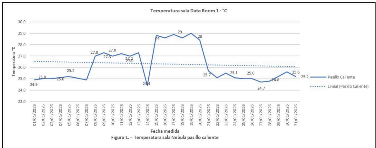
Figura 2 - Temperatura Sala Nebula
