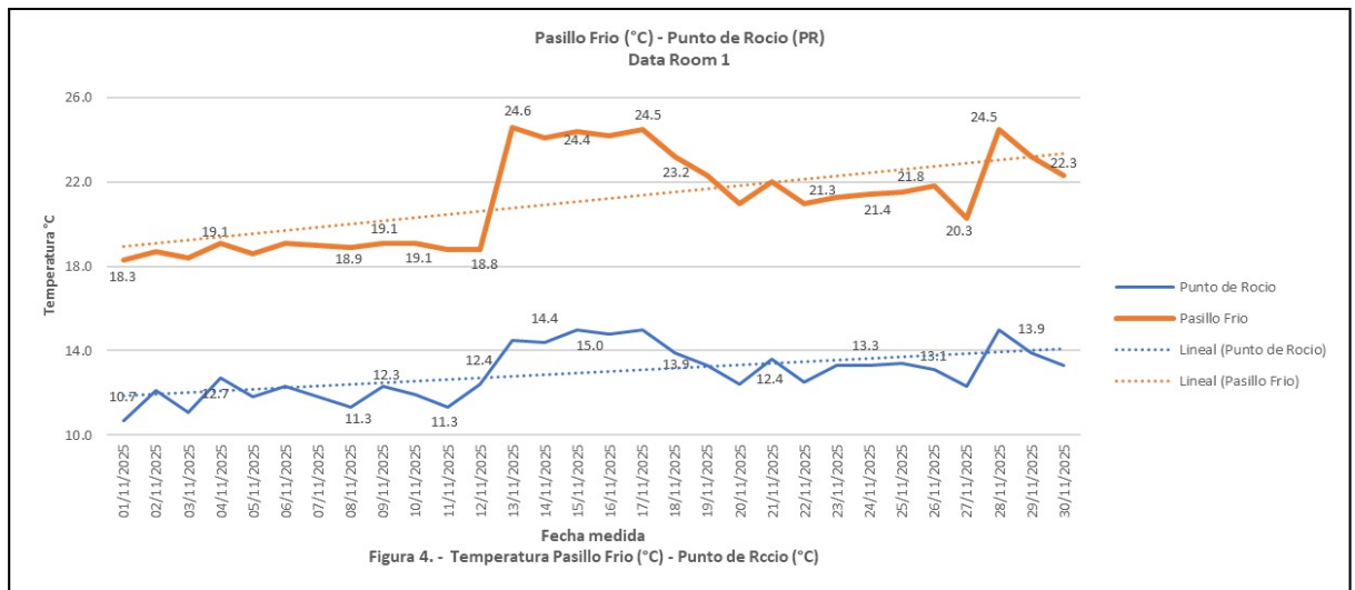
Figura 5 - Temperatura Pasillo Frio (°C) - Punto de Rocío (°C)
