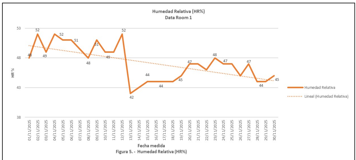
Figura 6 - Humedad Relativa (HR%)
