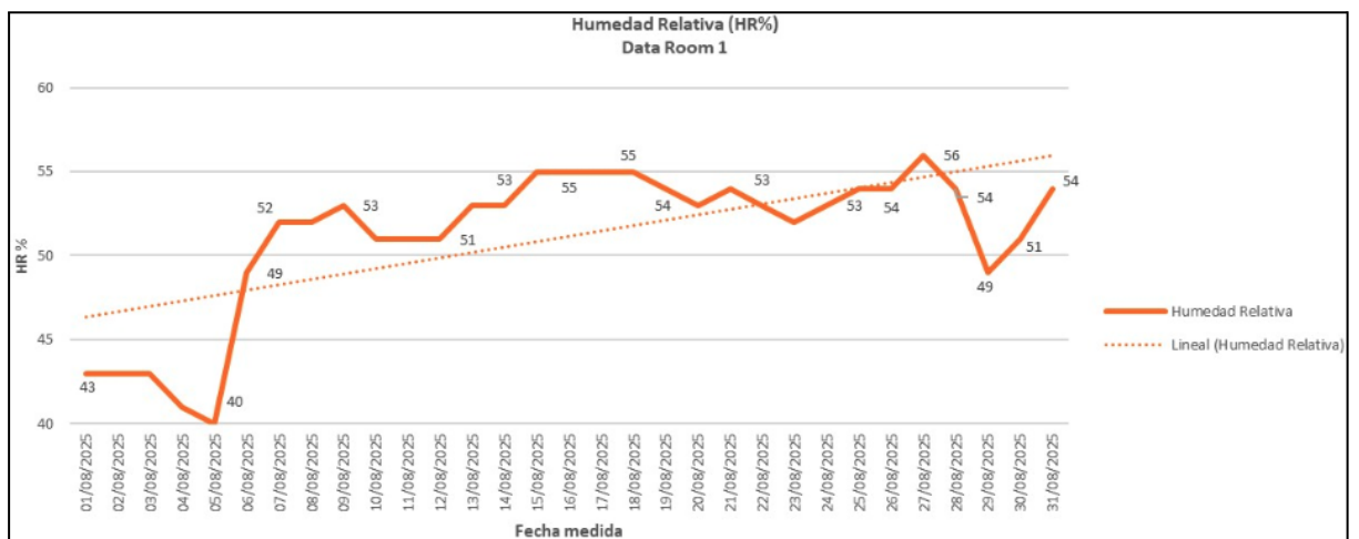
Figura 6 - Humedad Relativa (HR%)
