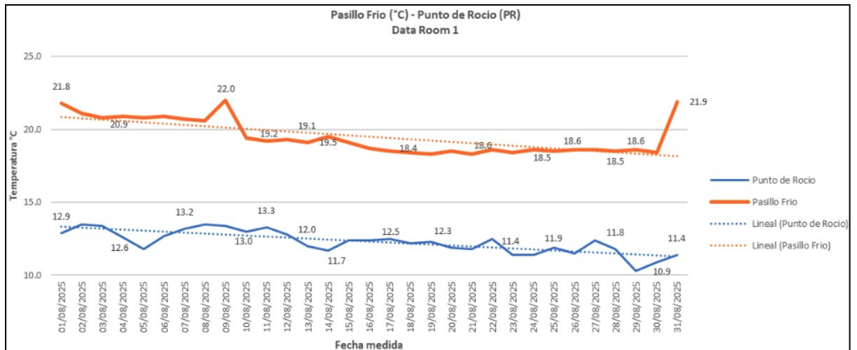
Figura 5 - Temperatura Pasillo Frio (°C) - Punto de Rocio (°C)
