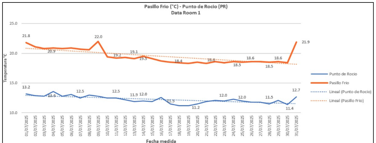
Figura 5 - Temperatura Pasillo Frio (°C) - Punto de Rocio (°C)
