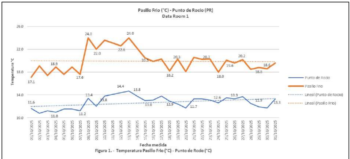
Figura 5 - Temperatura Pasillo Frío (°C) - Punto de Rocío (°C)
