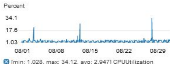
CPUUtilization-ETL-prod
