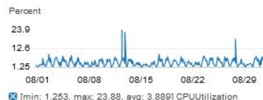
CPUUtilization-CapadeNegocio1-prod
