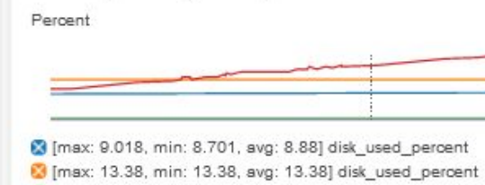
Disk-CapadeNegocio2-prod
