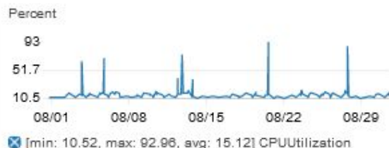
CPUUtilization-ServidorPROXY-prod
