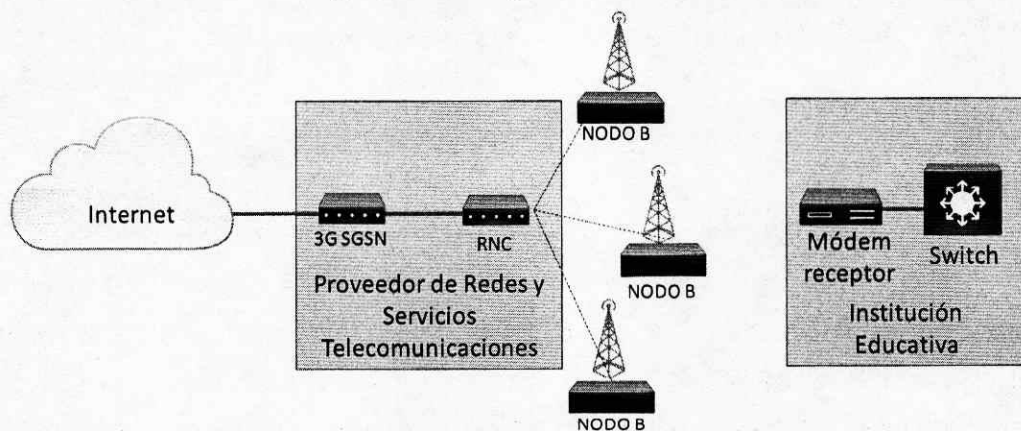
Figura 7. Tecnología de acceso radio Terrestre
