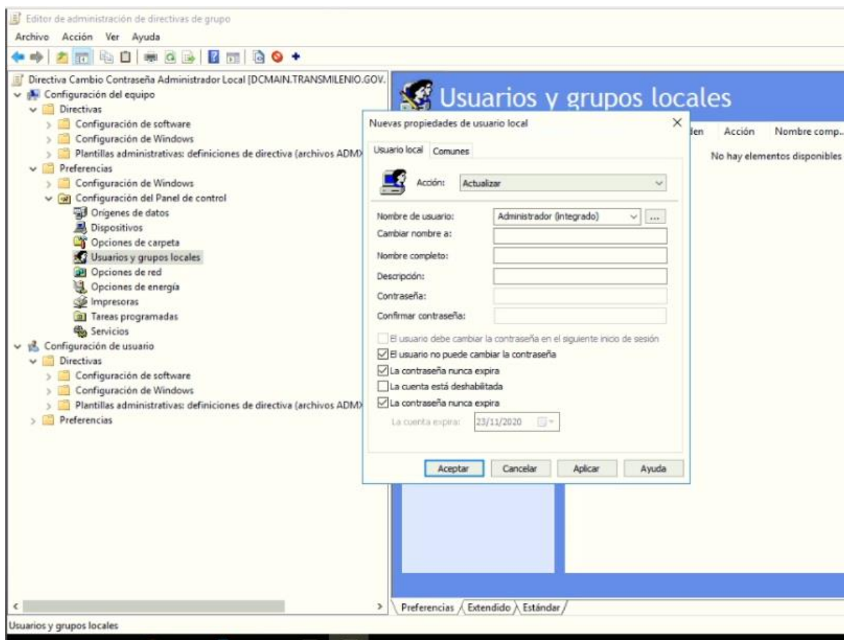
Ilustración 12 Cambio de password Administrador local de las maquinas del Dominio
