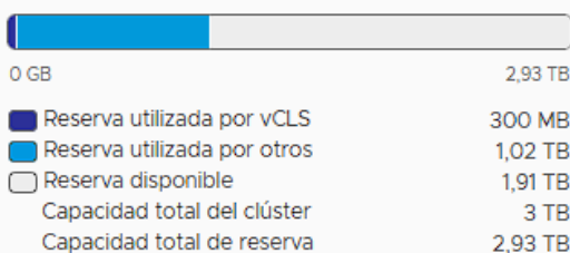
Figura 6. Consumo de memoria en Clúster de Aplicaciones.
