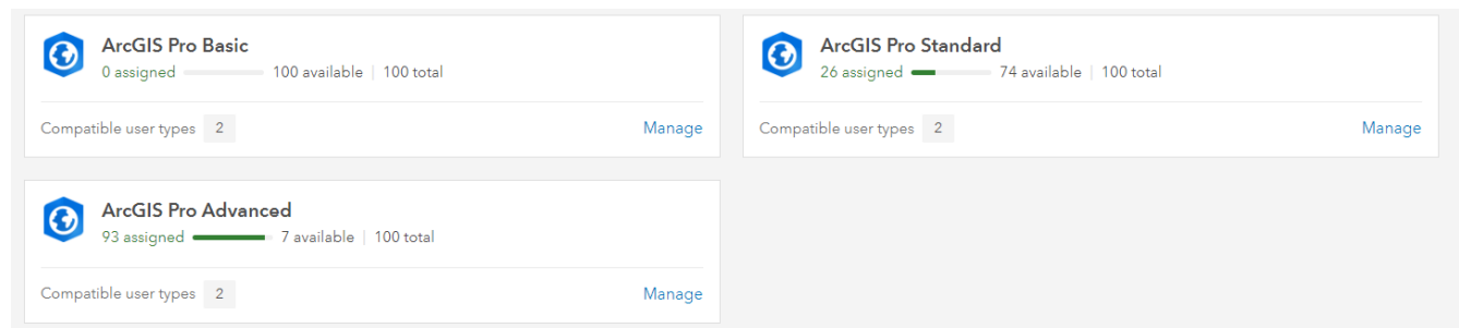
Gráfico 5. ArcGIS Pro
