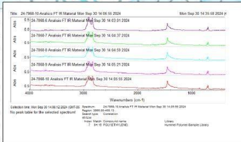
Gráfica Composición Análisis FTIR - Material
