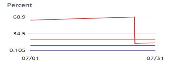
Disk-ServidorPROXY-prod
