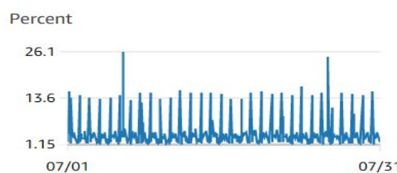
CPUUtilization-ETL-prod
