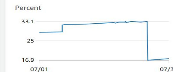
Disk-ETL-prod
