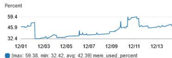
Memory-ServidorPROXY-prod
