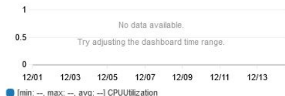
CPUUtilization-ServidorPROXY2-prod
