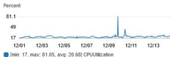
CPUUtilization-ServidorPROXY-prod
