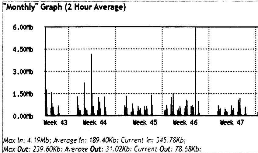
Fig39 Consumo y disponibilidad del canal mensual correspondiente al periodo 26 de octubre al 25 de noviembre.
