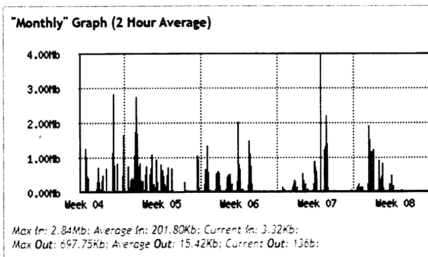
Fig21 Consumo y disponibilidad del canal mensual correspondiente al periodo del 22 de enero al 21 de febrero del 2024.
