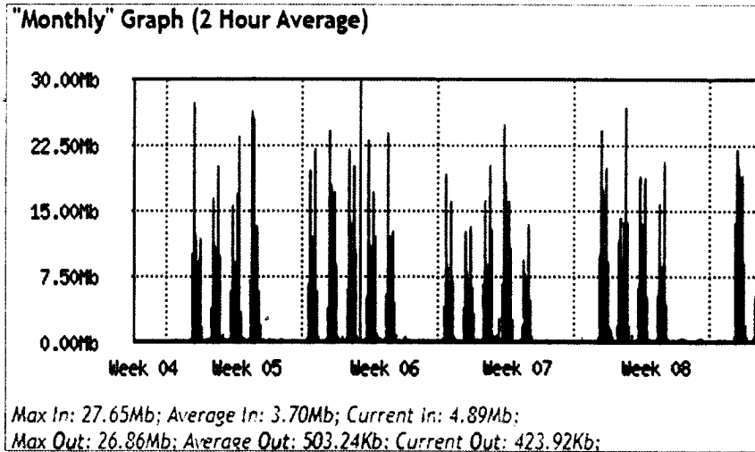
Fig55 Consumo y disponibilidad del canal mensual correspondiente al periodo del 22 de enero al 21 de febrero del 2024.
