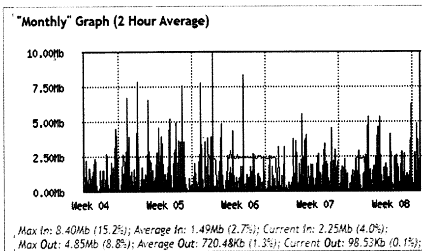
Fig158 Consumo y disponibilidad del canal mensual correspondiente al periodo del 22 de enero al 21 de febrero del 2024.
