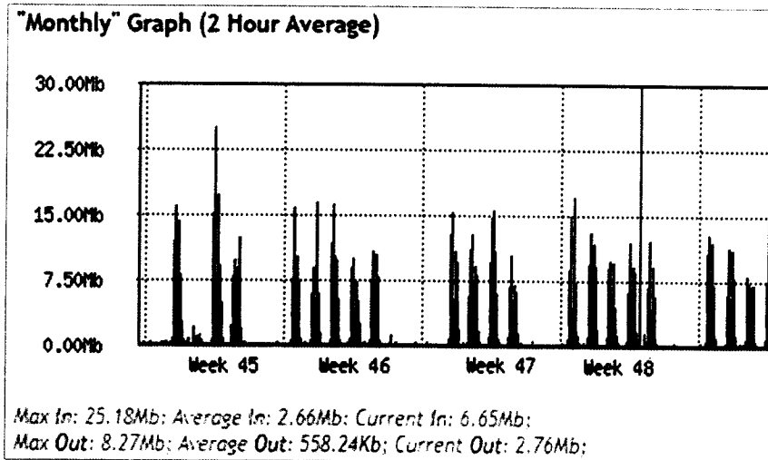
Fig144 Consumo y disponibilidad del canal mensual correspondiente al periodo 11 al 30 de noviembre
