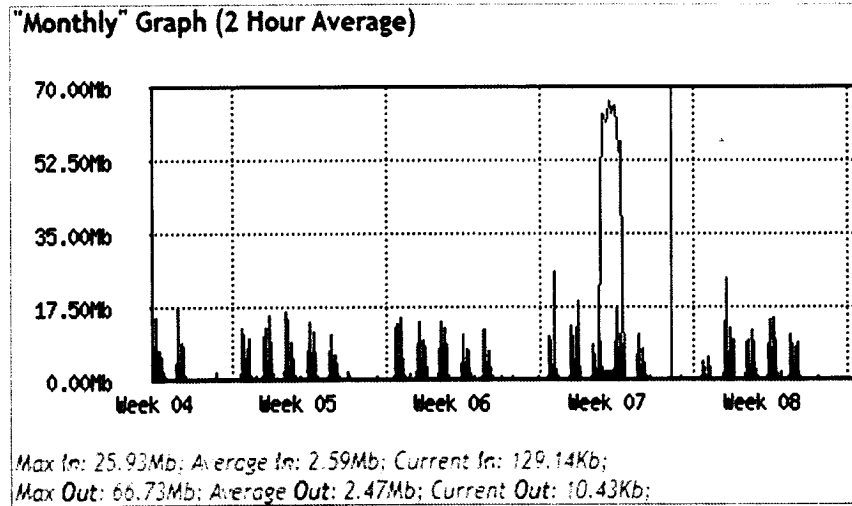
Fig102 Consumo y disponibilidad del canal mensual correspondiente al periodo del 22 de enero al 21 de febrero del 2024.
