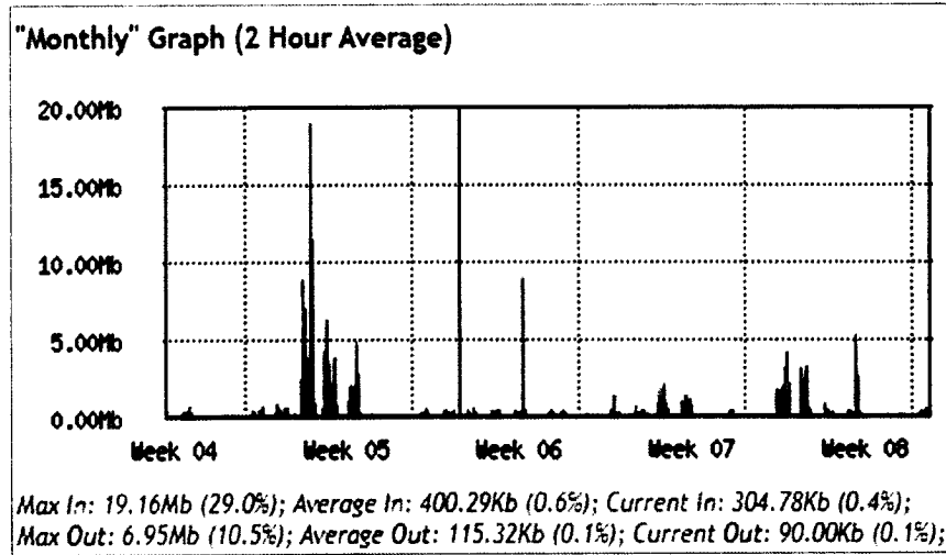
Fig7 Consumo y disponibilidad del canal mensual correspondiente al periodo del 22 de enero al 21 de febrero del 2024.
