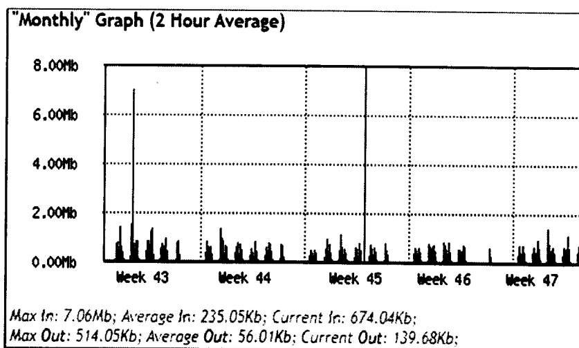
Fig66 Consumo y disponibilidad del canal mensual correspondiente al periodo 26 de octubre al 25 de noviembre.
