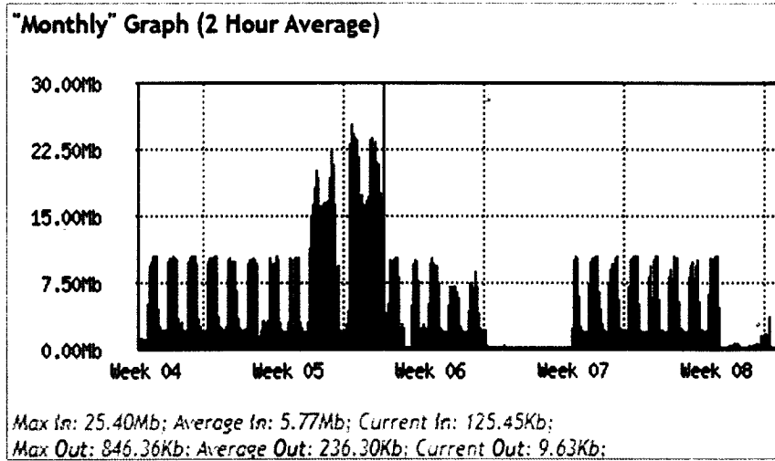
Fig143 Consumo y disponibilidad del canal mensual correspondiente al periodo del 22 de enero al 21 de febrero del 2024.
