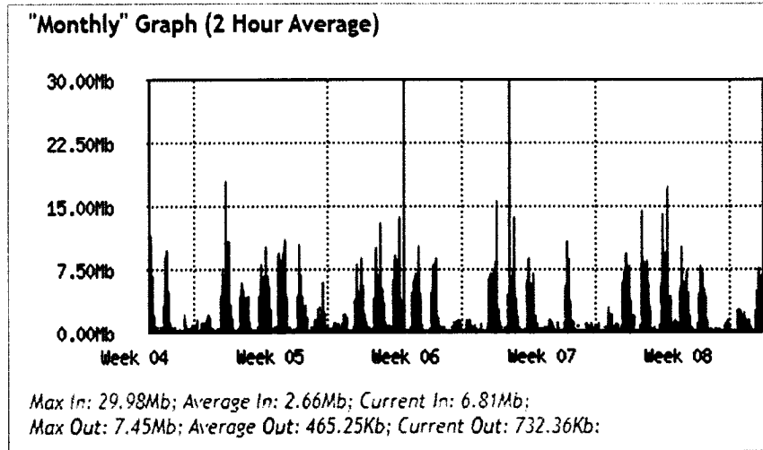
Fig135 Consumo y disponibilidad del canal mensual correspondiente al periodo del 22 de enero al 21 de febrero del 2024.
