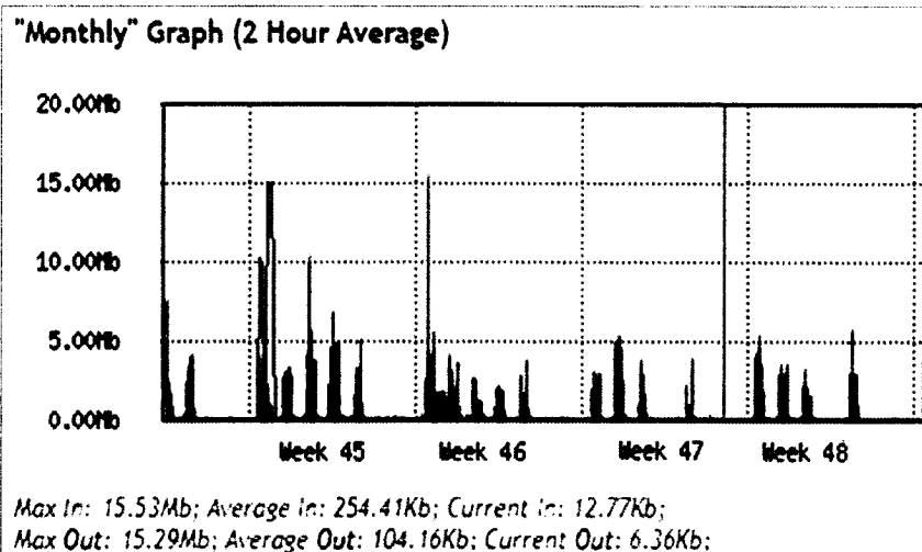
Fig141 Consumo y disponibilidad del canal mensual correspondiente al periodo 11 al 30 de noviembre
