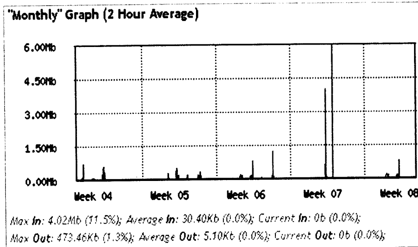
Fig182 Consumo y disponibilidad del canal mensual correspondiente al periodo del 22 de enero al 21 de febrero del 2024.
