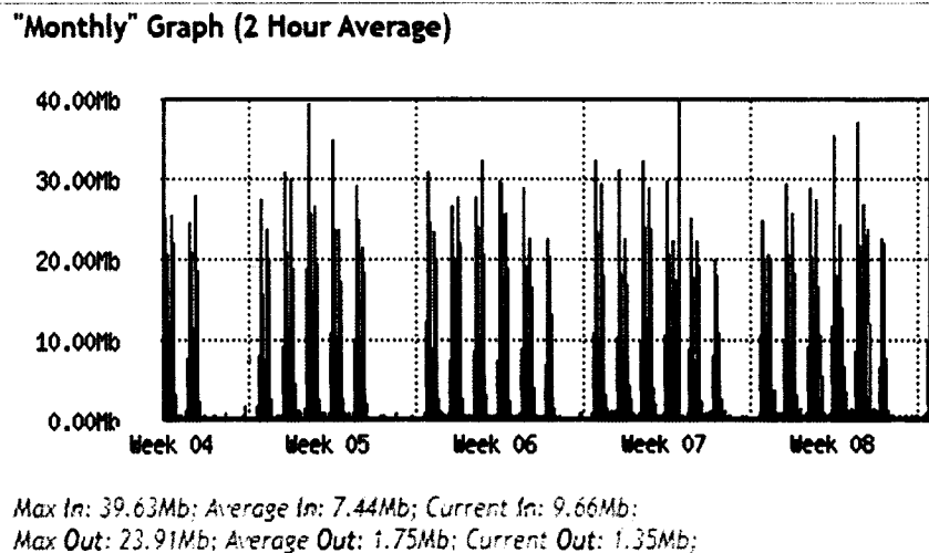
Fig60 Consumo y disponibilidad del canal mensual correspondiente al periodo del 22 de enero al 21 de febrero del 2024.
