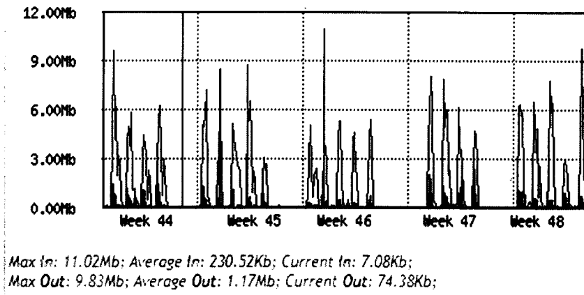
Fig31 Consumo y disponibilidad del canal mensual correspondiente al periodo 30 de octubre al 29 de noviembre.
