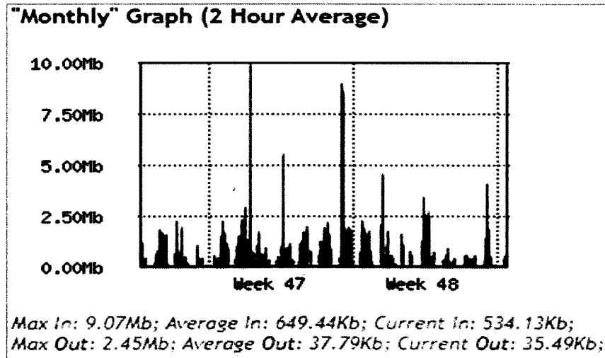
Fig26 Consumo y disponibilidad del canal mensual correspondiente al periodo 20 al 30 de noviembre.
