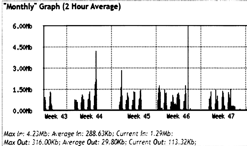
Fig38 Consumo y disponibilidad del canal mensual correspondiente al periodo 26 de octubre al 25 de noviembre.
