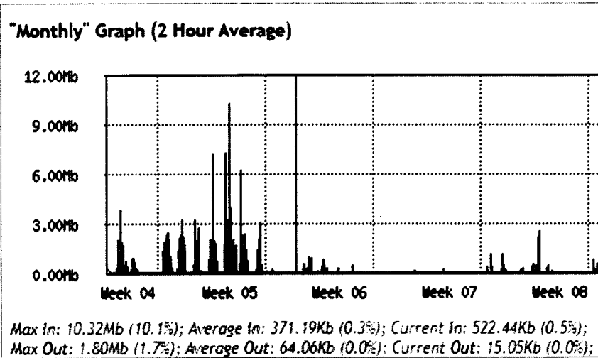
Fig117 Consumo y disponibilidad del canal mensual correspondiente al periodo del 22 de enero al 21 de febrero del 2024.
