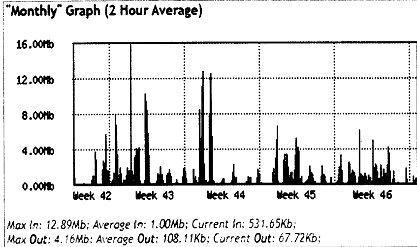
Fig8 Consumo y disponibilidad del canal mensual correspondiente al periodo 20 de octubre al 19 de noviembre.
