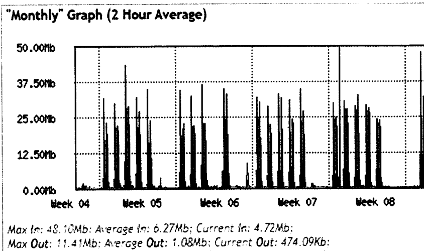
Fig106 Consumo y disponibilidad del canal mensual correspondiente al periodo del 22 de enero al 21 de febrero del 2024.
