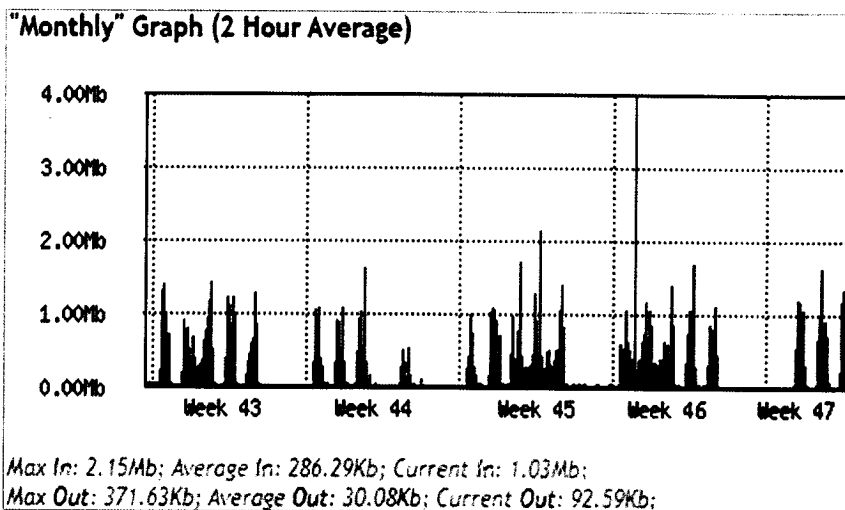
Fig45 Consumo y disponibilidad del canal mensual correspondiente al periodo 26 de octubre al 25 de noviembre.
