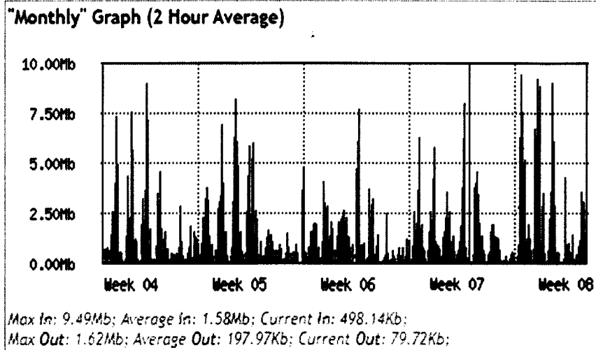
Fig161 Consumo y disponibilidad del canal mensual correspondiente al periodo del 22 de enero al 21 de febrero del 2024.
