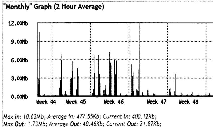
Fig77 Consumo y disponibilidad del canal mensual correspondiente al periodo 30 de octubre al 29 de noviembre.
