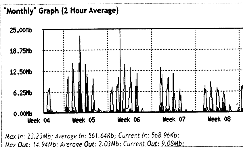
Fig144 Consumo y disponibilidad del canal mensual correspondiente al periodo del 22 de enero al 21 de febrero del 2024.
