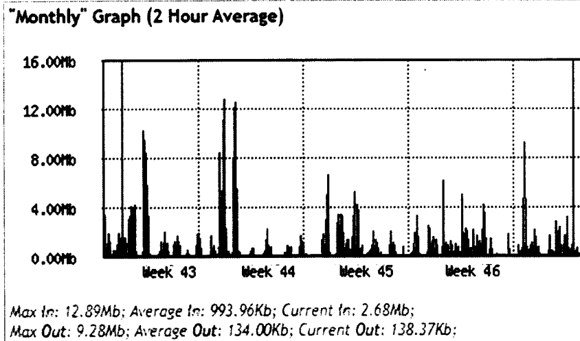
Fig10 Consumo y disponibilidad del canal mensual correspondiente al periodo 21 de octubre al 20 de noviembre.
