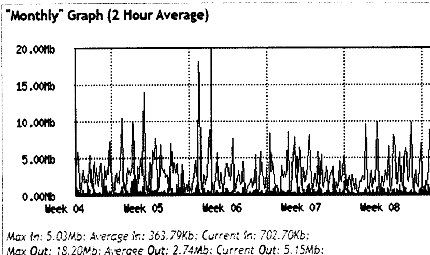
Fig176 Consumo y disponibilidad del canal mensual correspondiente al periodo del 22 de enero al 21 de febrero del 2024.
