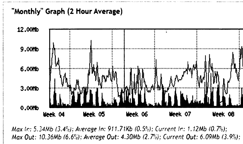
Fig97 Consumo y disponibilidad del canal mensual correspondiente al periodo del 22 de enero al 21 de febrero del 2024.
