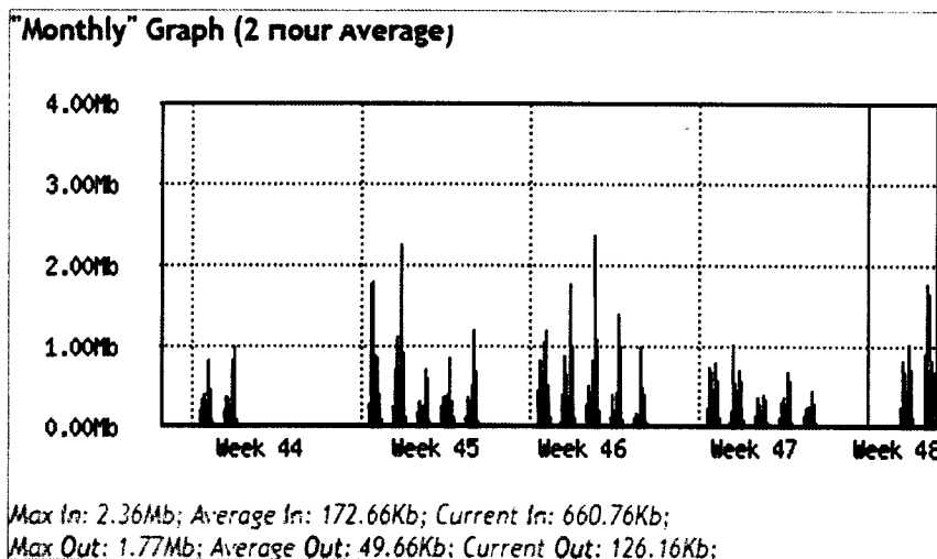
Fig33 Consumo y disponibilidad del canal mensual correspondiente al periodo 30 de octubre al 29 de noviembre.
