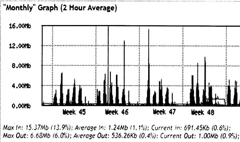
Fig178 Consumo y disponibilidad del canal mensual correspondiente al periodo 7 al 30 de noviembre
