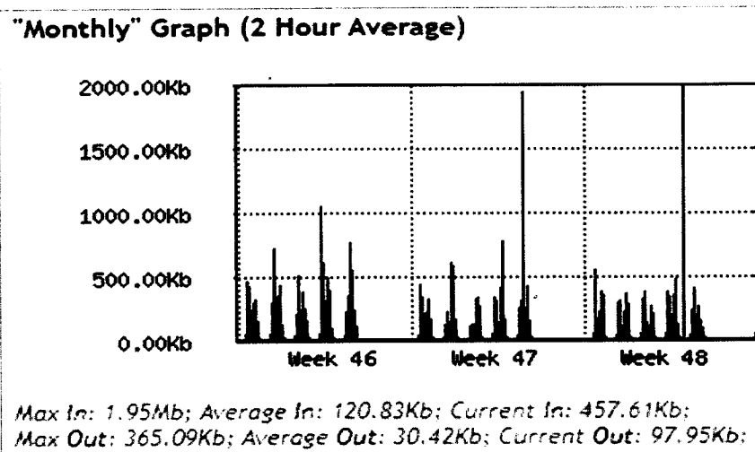
Fig105 Consumo y disponibilidad del canal mensual correspondiente al periodo 19 al 30 de noviembre.
