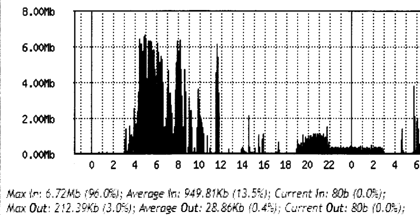
Fig183 Consumo y disponibilidad del canal correspondiente al día 30 de noviembre.
