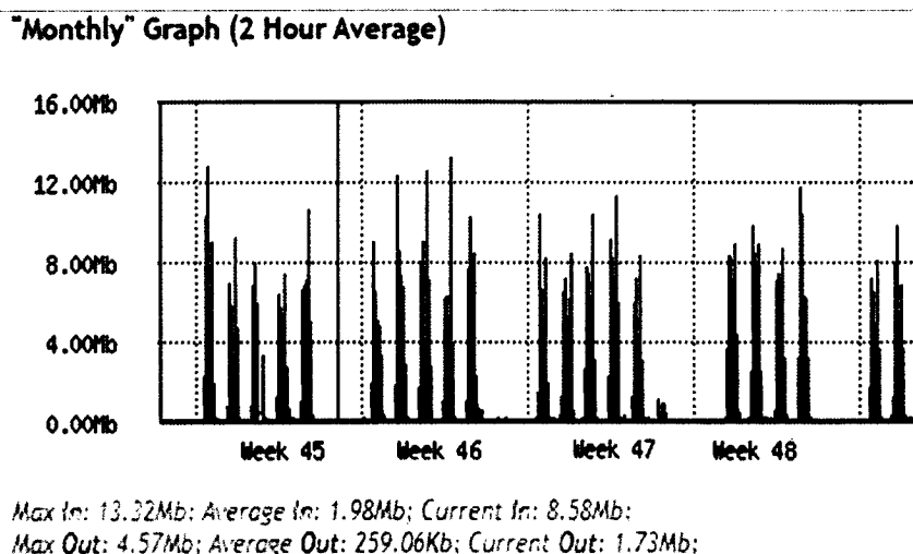
Fig181 Consumo y disponibilidad del canal mensual correspondiente al periodo 11 al 30 de noviembre
