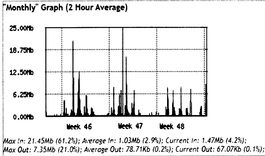
Fig46 Consumo y disponibilidad del canal mensual correspondiente al periodo 16 al 30 de noviembre
