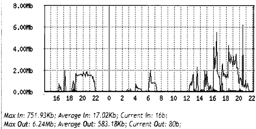
Fig12 Consumo y disponibilidad del canal correspondiente al día 30 de noviembre.
