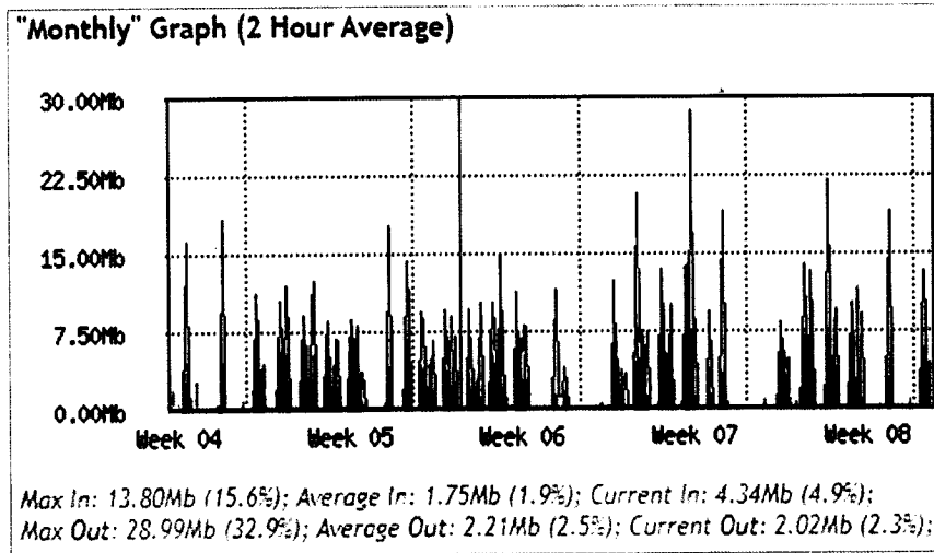
Fig172 Consumo y disponibilidad del canal mensual correspondiente al periodo del 22 de enero al 21 de febrero del 2024.
