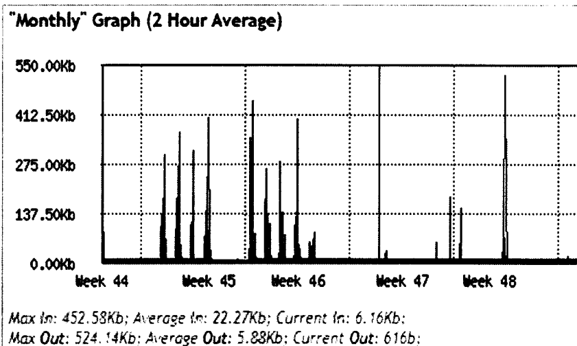
Fig87 Consumo y disponibilidad del canal mensual correspondiente al periodo 1 al 30 de noviembre.
