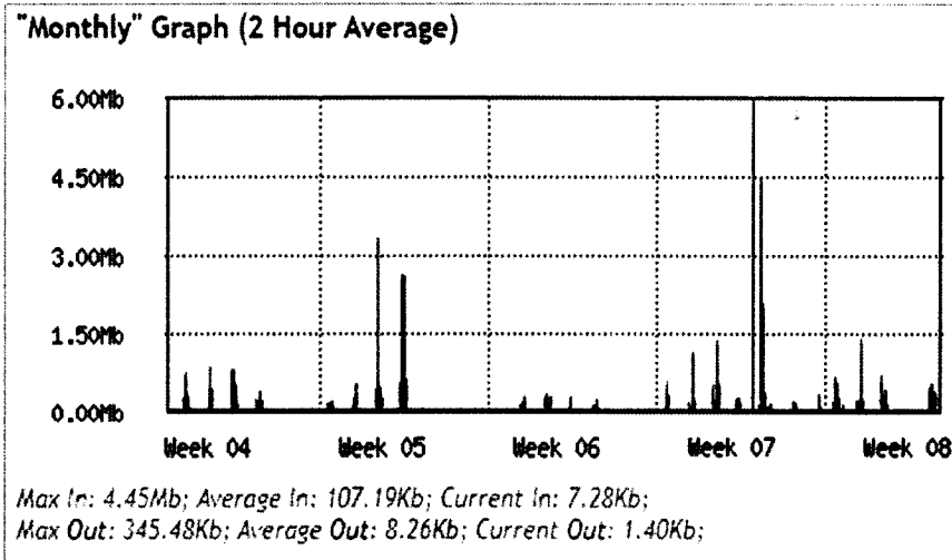
Fig16 Consumo y disponibilidad del canal mensual correspondiente al periodo del 22 de enero al 21 de febrero del 2024.
