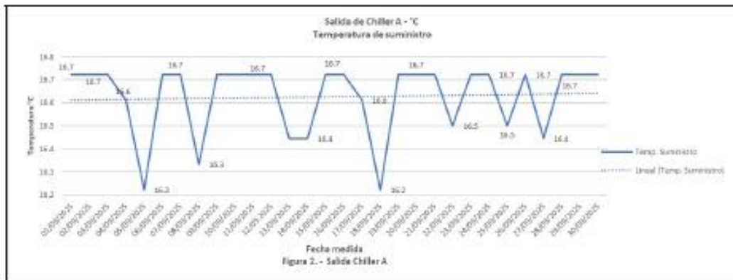
Figura 3 - Salida chiller A
