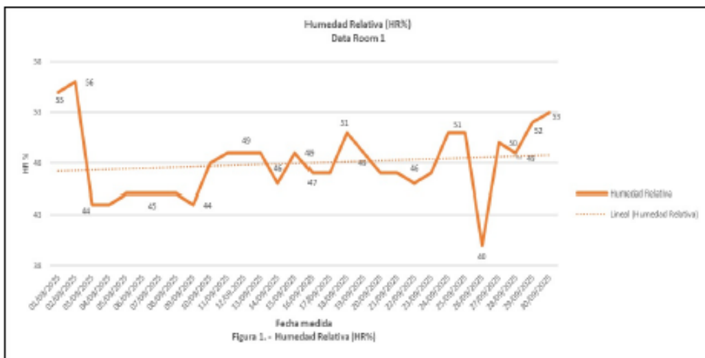
Figura 6 - Humedad Relativa (HR%)
