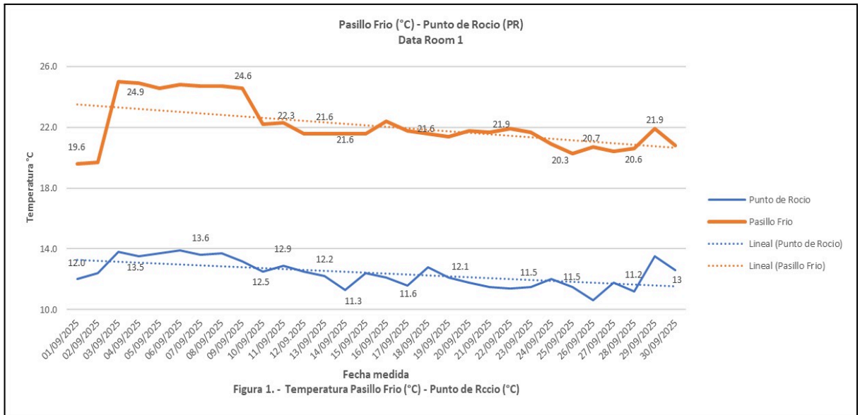
Figura 5 - Temperatura Pasillo Frío (°C) - Punto de Rocío (°C)
