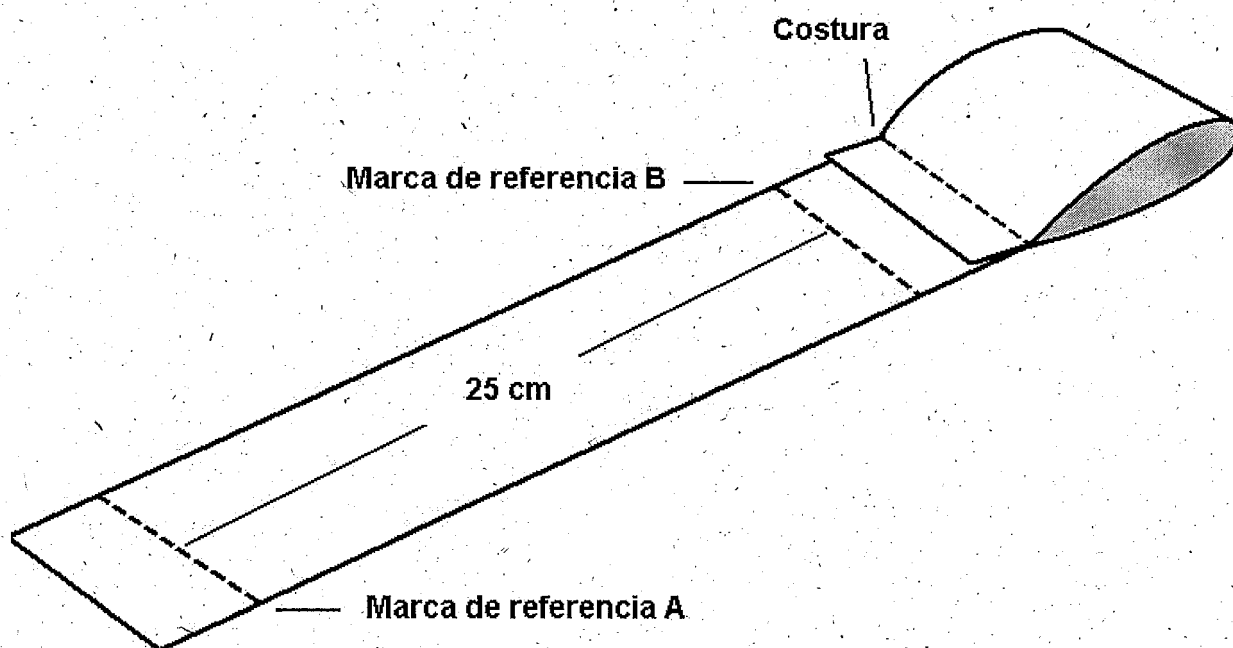
Figura 3. Probeta de elongación de la tela.
