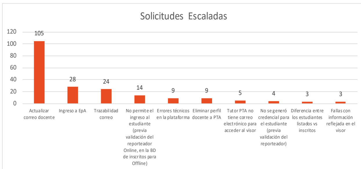
Ilustración 13 Solicitudes escaladas
