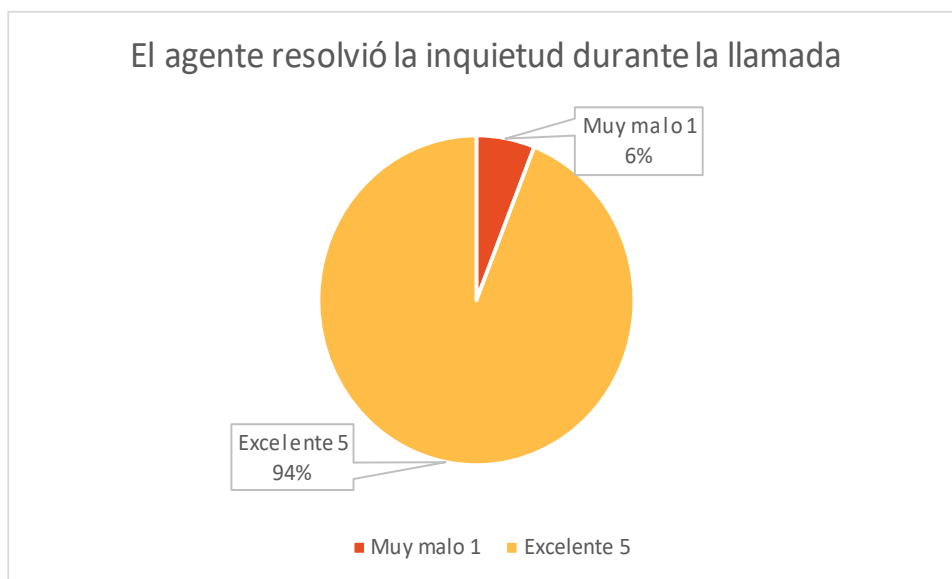
Ilustración 26 análisis pregunta 2
